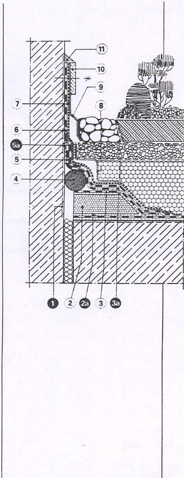
WIROBIT-Abdichtung 2-lagig
